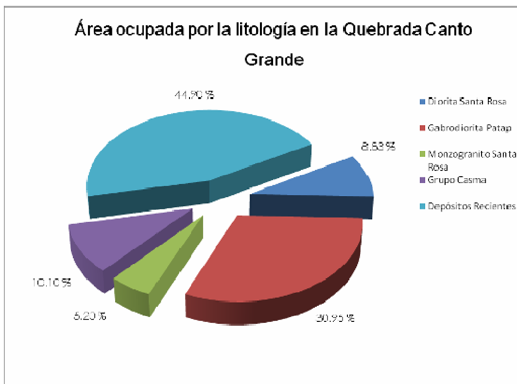
Gráfico 5.1 Litología de la Quebrada Canto Grande
