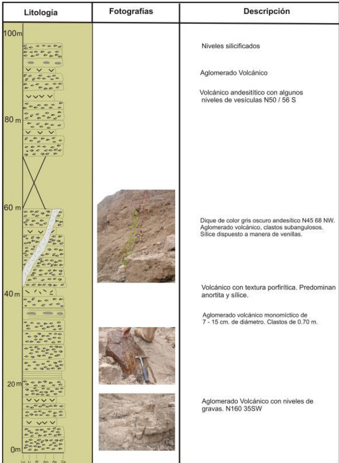
Gráfico 4.2 Columna Estratigráfica de la parte alta de la Quebrada Canto Grande. Coordenadas (N 8603366 E288688)
