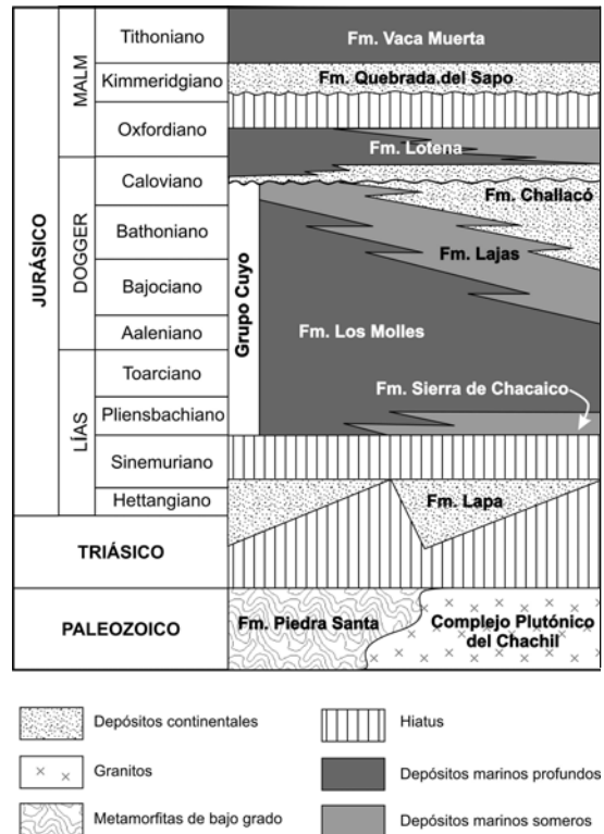
FIG. 4. Cuadro cronoestratigráfico pre-cretácico para el sector sur de la Cuenca Neuquina.
