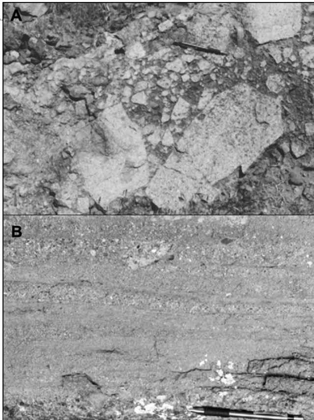
FIG. 8. La sección inferior del 'sin-rift' en la sierra de Chacaico. A. Brechas gruesas volcánicas (autobrecha). Sección Antinao. B. Facies arenosas gruesas a medianas con estratificación horizontal interpretadas como depósitos de flujos hiperconcentrados. Sección inferior del perfil Currú Charahuilla.
