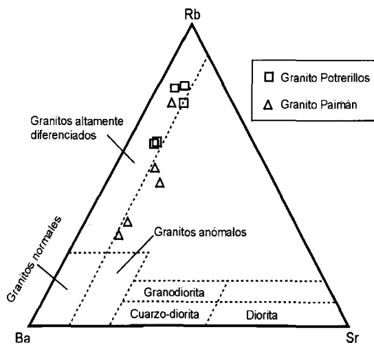
FIG. 9. Diagrama triangular Rb-Ba-Sr de El Bouseily y El Sokkary (1975) para los granitos Paimán y Potrerillos.
