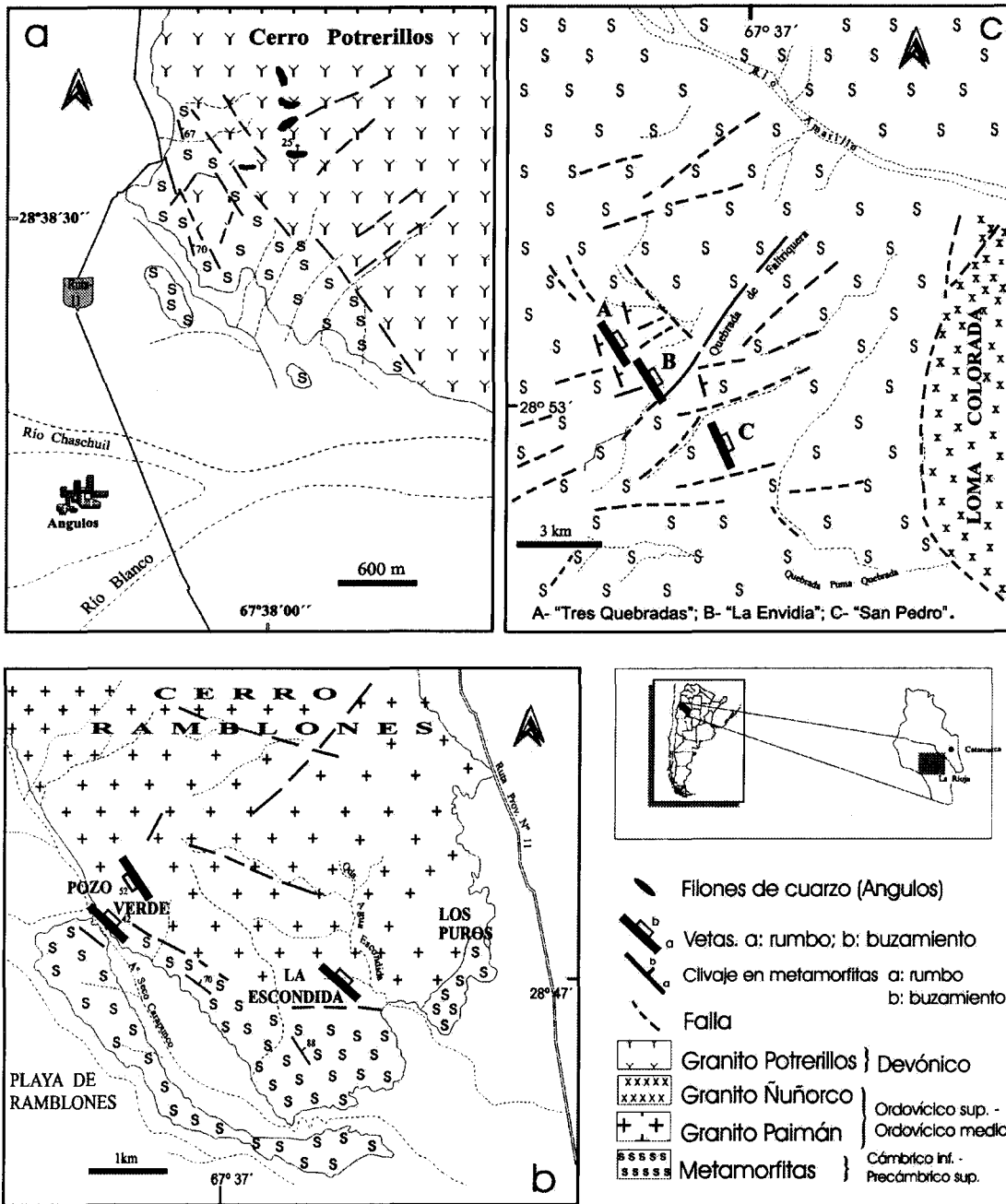
FIG. 4. Geología local de cada área mineralizada. a) Ángulos (modificado de Sardi y Rossi de Toselli, 1999); b) Ramblones; c) Faltriguera.
