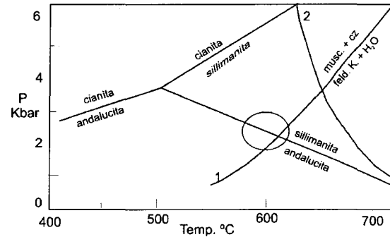
FIG. 6. Diagrama de presión-temperatura. El círculo representa las condiciones P-T de formación del yacimiento Los Puros del área Ramblones. Curva 1: muscovita-cuarzo de Helgeson et al. (1978). Curva 2: fusión albita-feldespato potásico-cuarzo-agua+líquido de Thompson y Tracy (1979). Curva de estabilidad de aluminosilicatos de Holdaway (1971).
