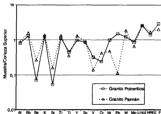
FIG. 3. Normalización de los Granitos Paimán y Potrerillos (valores promedio) a corteza superior según valores de Wedephol (1995).
