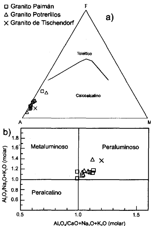
FIG. 2. Diagramas geoquímicos para los Granitos Paimán y Potrerillos. a) diagrama triangular AFM (A=Na 2 O+K 2 O; F=FeO+Fe 2 O 3 ; M=MgO) con límite de Irvine y Baragar (1971); b) diagrama ortogonal de aluminosidad de Maniar y Piccoli (1989).
