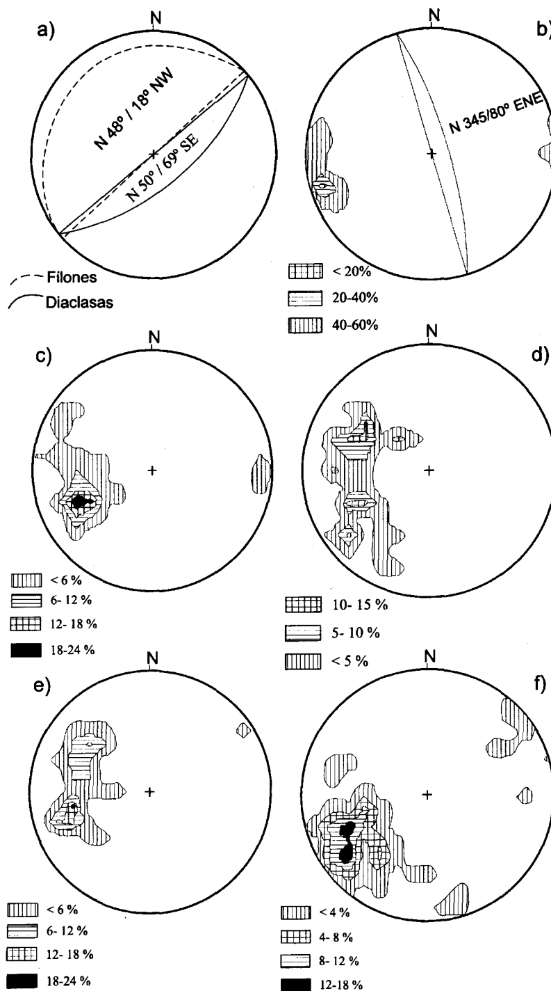
FIG. 5. Falsilla equiareal de Schmidt, hemisfera inferior, en la que se proyectan valores de rumbo y buzamiento de diferentes planos estructurales. a) plano promedio de las diaclasas del Granito Potrerillos y de los filones del área Angulos; b) plano representativo de las principales estructuras en la mina Los Puros del área Ramblones, especialmente esquistosidad; c, d y e) rumbo e inclinación de las vetas del área de Faltriquera, mina Tres Quebradas, La Envidia y San Pedro, respectivamente; f) clivaje de las metamorfitas de la Formación Negro Peinado en el área de Faltriquera.
