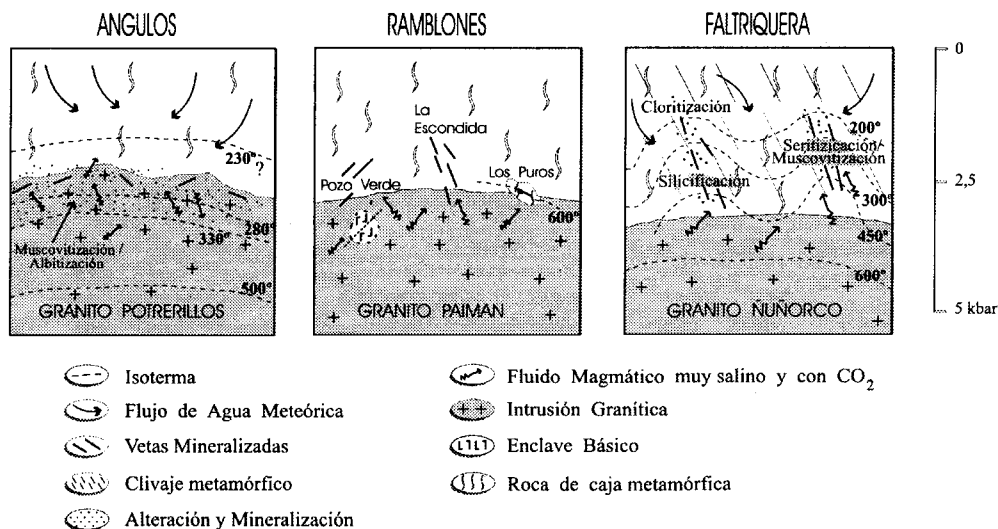
FIG. 11. Esquema interpretativo de la génesis de los yacimientos de Ángulos, Ramblones y Faltriquera.
