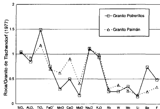
FIG. 10. Normalización de los Granitos Paimán y Potrerillos con el especializado de Tischendorf (1977) (valores promedio).
