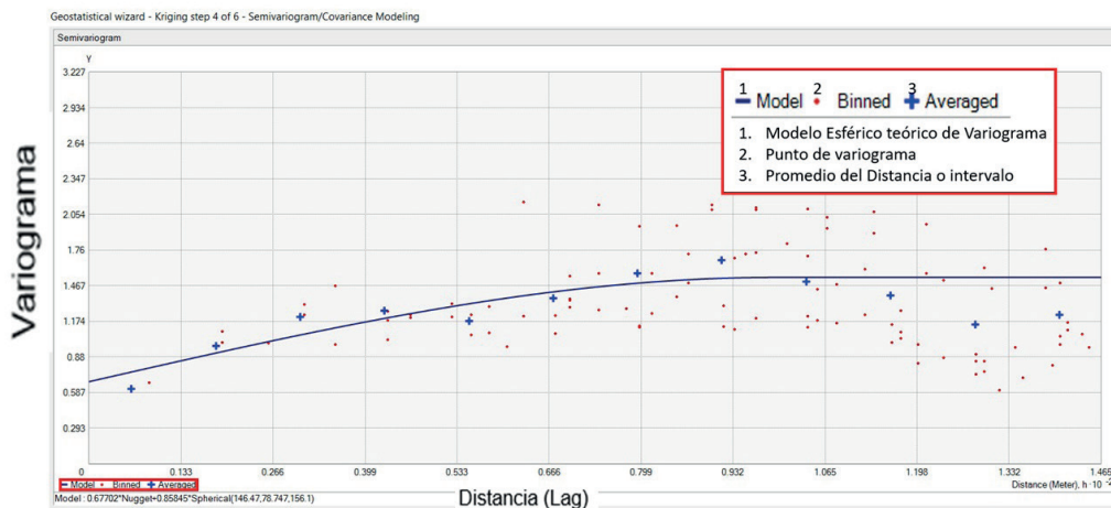
Figura N° 03. Variograma del Au en dirección 100°.
