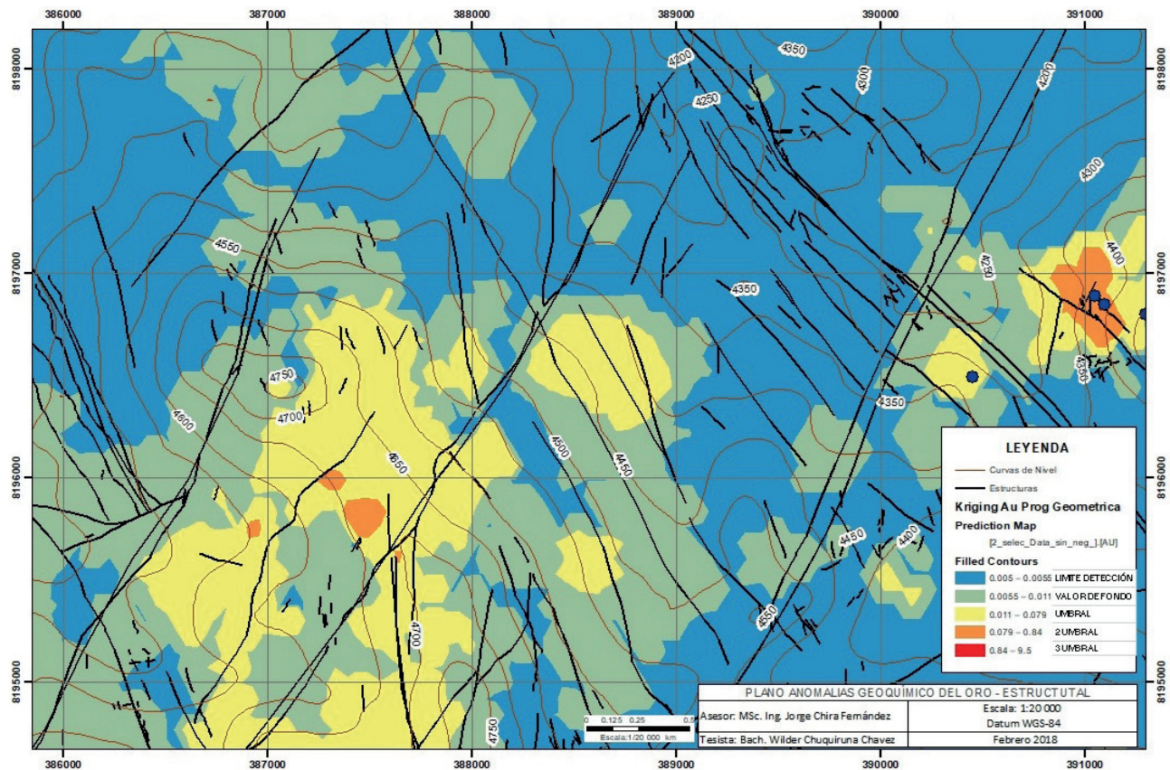
Figura N° 08. Modelo de anomalía geoquímica, Kriging del Au y lineamientos estructurales
