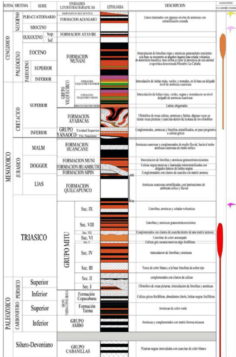
Figura 4 Columna estratigráfica generalizada de la cuenca del Titicaca (tomado de Acosta, 2001).
