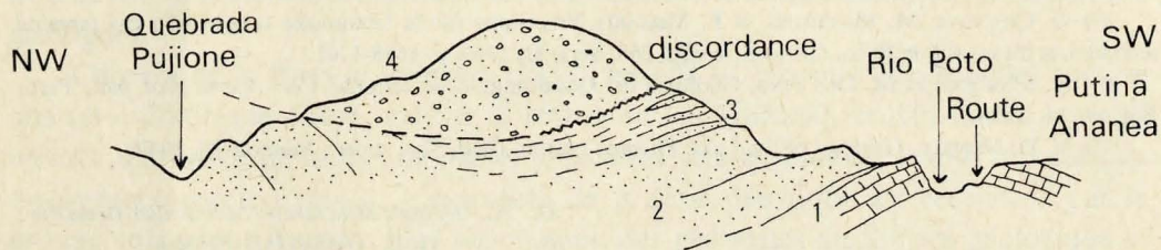
Fig. 2. — Coupe de la Quebrada region. 1. F. Copacabana (calcaire) ; 2. F. Cotacucho (grès rouges) ; 3. F. Vilquechico (Pélites grises et grès gris) ; 4. Gr. Puno (Conglomérats bréchiques).
