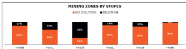
Figura 12: Porcentaje de la dilución por tajo
