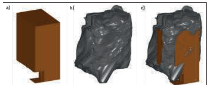
Figura 6: a) Solido 3D del diseño del tajo b) Solido 3D del levantamiento topográfico del tajo vacío. c) contraste entre el sólido 3D diseñado y el sólido 3D levantado
