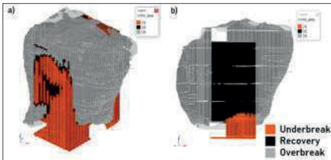
Figura 7: a) Vista isométrica del levantamiento topográfico de un tajo clasificado por recuperación, overbrake y underbrake. b) Sección del levantamiento topográfico de un tajo finalizado clasificado por recuperación, overbrake y underbrake.
