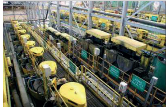
Figura 5: Tanques de flotación de la planta de beneficio de Cerro Lindo
