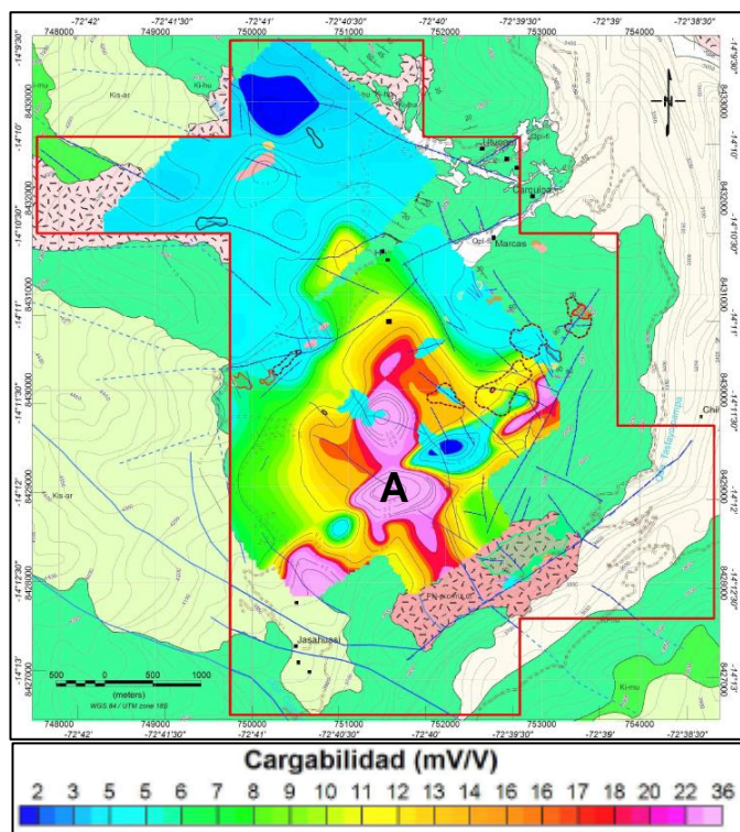
Figura 4. Cargabilidad a una profundidad de 300 m.
