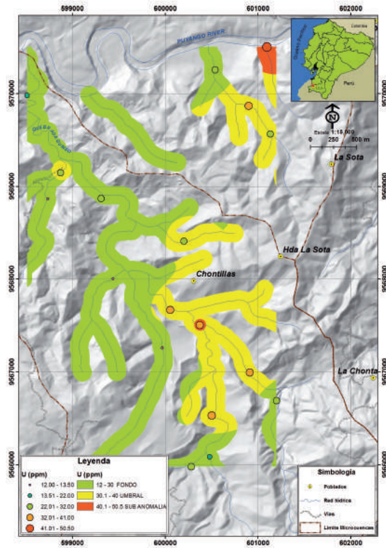
Figura 10. Mapas geoquímicos de: A. V, B. Zn y C. U respectivamente en la subcuenca Guineo.
