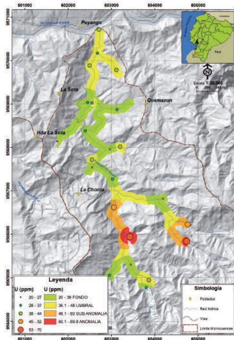
Figura 8. Mapas geoquímicos de: A. V, B. Zn y C. U respectivamente en la subcuenca Chirimoyo.
