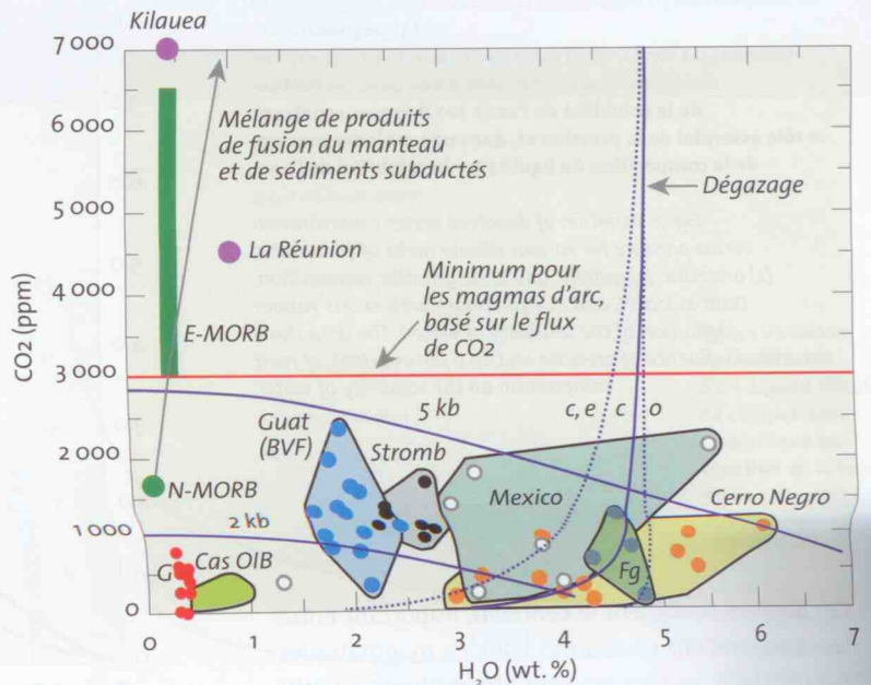
Fig. 1 : Compilation des données de concentration en eau et en CO_2 dans les inclusions vitreuses des basaltes. Données des volcans d'arc d'Amérique Centrale (Fuego, Fg ; Cerro Negro ; Guatemala en arrière du front volcanique, Guat BVF), de la ceinture volcanique trans-mexicaine (Mexico), du Stromboli (Stromb) et du Galunggung (G). À titre de comparaison, les données pour les basaltes océaniques (MORB, point et rectangle), et pour le Kilauea, La Réunion et un basalte de type île océanique de la chaîne des Cascades (Cas OIB) sont figurées.
