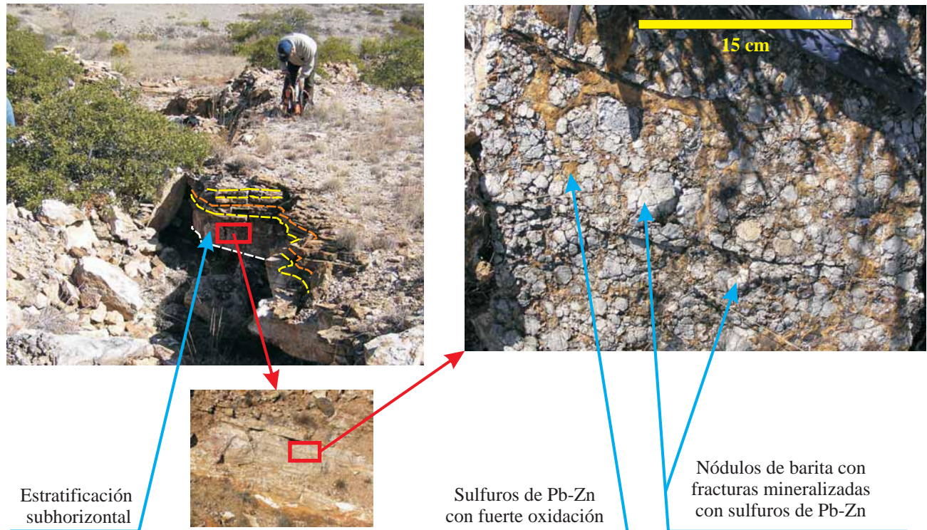
Figura 6. Fotografías mostrando el carácter estratoligado de la mineralización y la textura en nódulos de la barita (derivada posiblemente del reemplazamiento de nódulos de yeso o anhidrita) en los yacimientos de Pb-Zn-barita de la zona de Berrendos, Coahuila.
