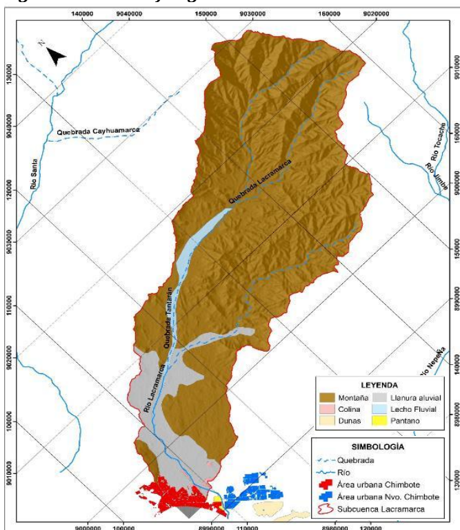
Figura 01. Geomorfológica de la subcuenca
