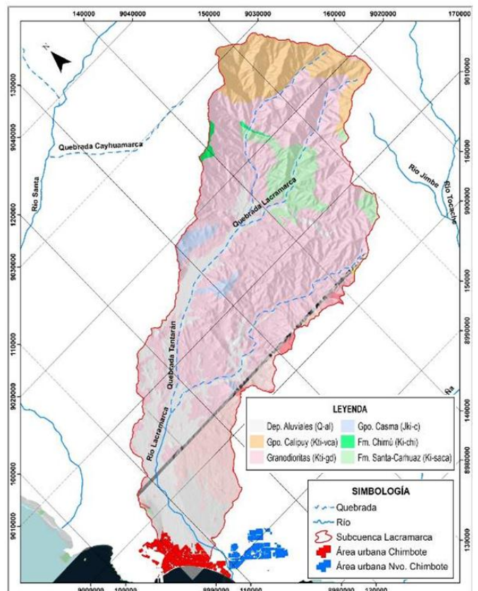
Figura 02. Geología de la subcuenca Lacramarca
