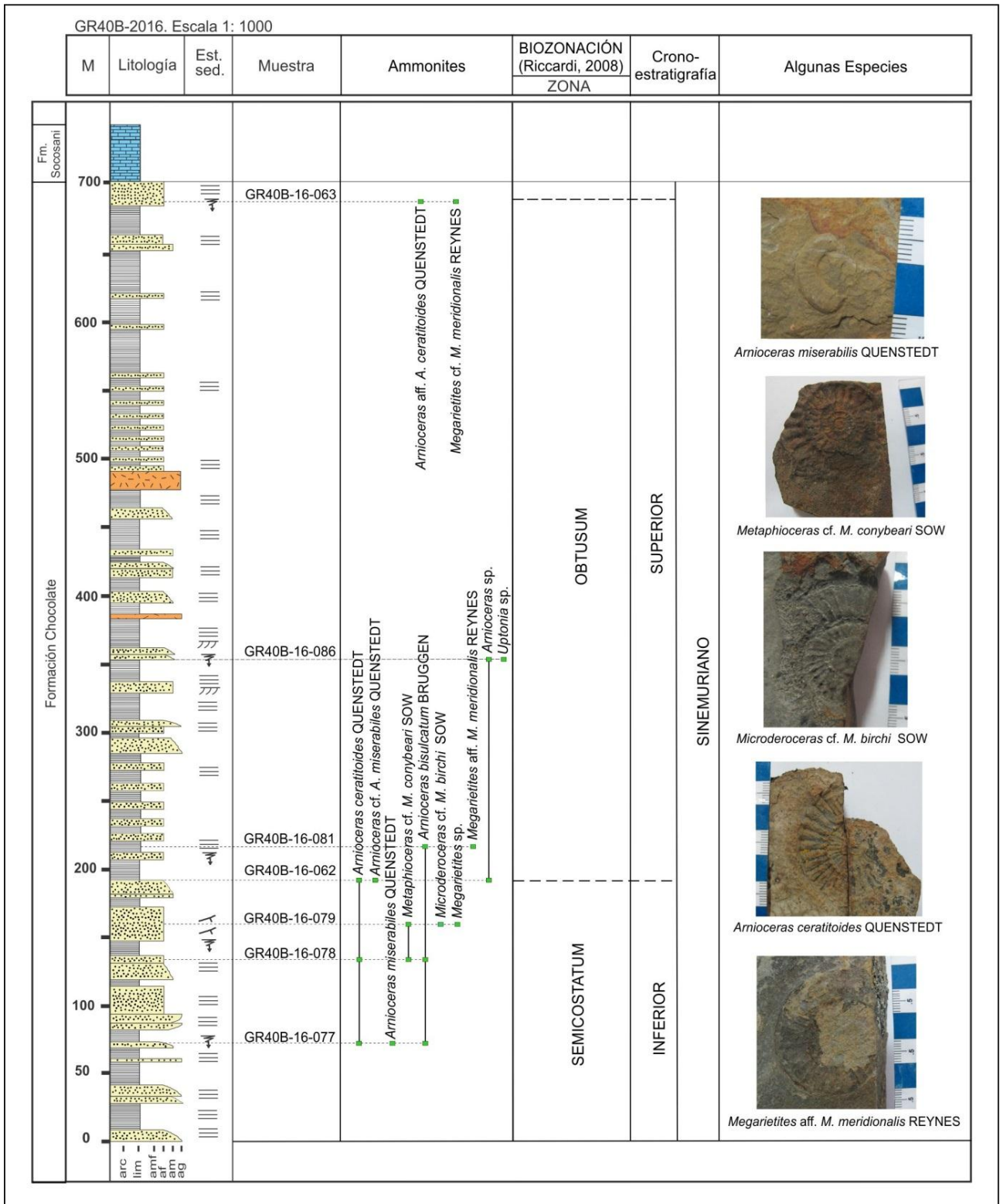
Figura 3. Columna lito-bioestratigráfica en el cerro Pariamocco.
