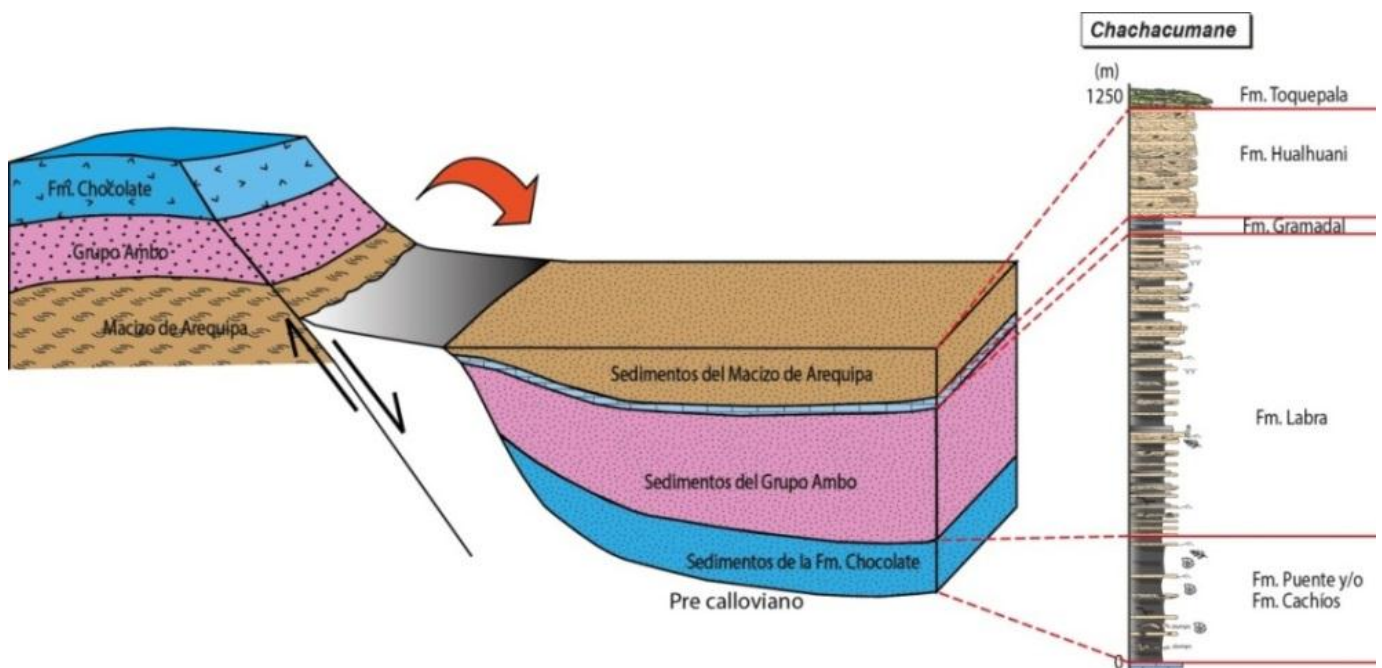
Figura 5. Modelo simplificado de procedencia sedimentaria de la cuenca Arequipa en Tacna.
