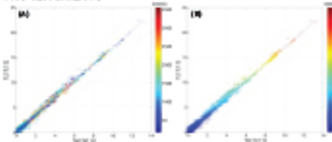
Figura 4.- Curvas de velocidad de ondas P y S para los sismos de la zona volcánica de los volcanes Misti y Chachani, se ve el estado de las estaciones sísmicas en el momento de la configuración de 2005 y 2012.
