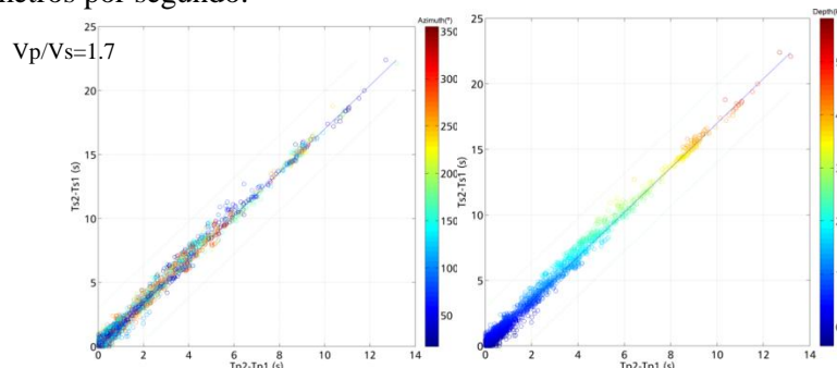
Figura 2.-Curva de Wadatti obtenida para los eventos sísmicos registrados en la campaña sísmica 2011 y 2012, mostrando la relación de velocidades en función A) del azimut y B) la profundidad como color.
