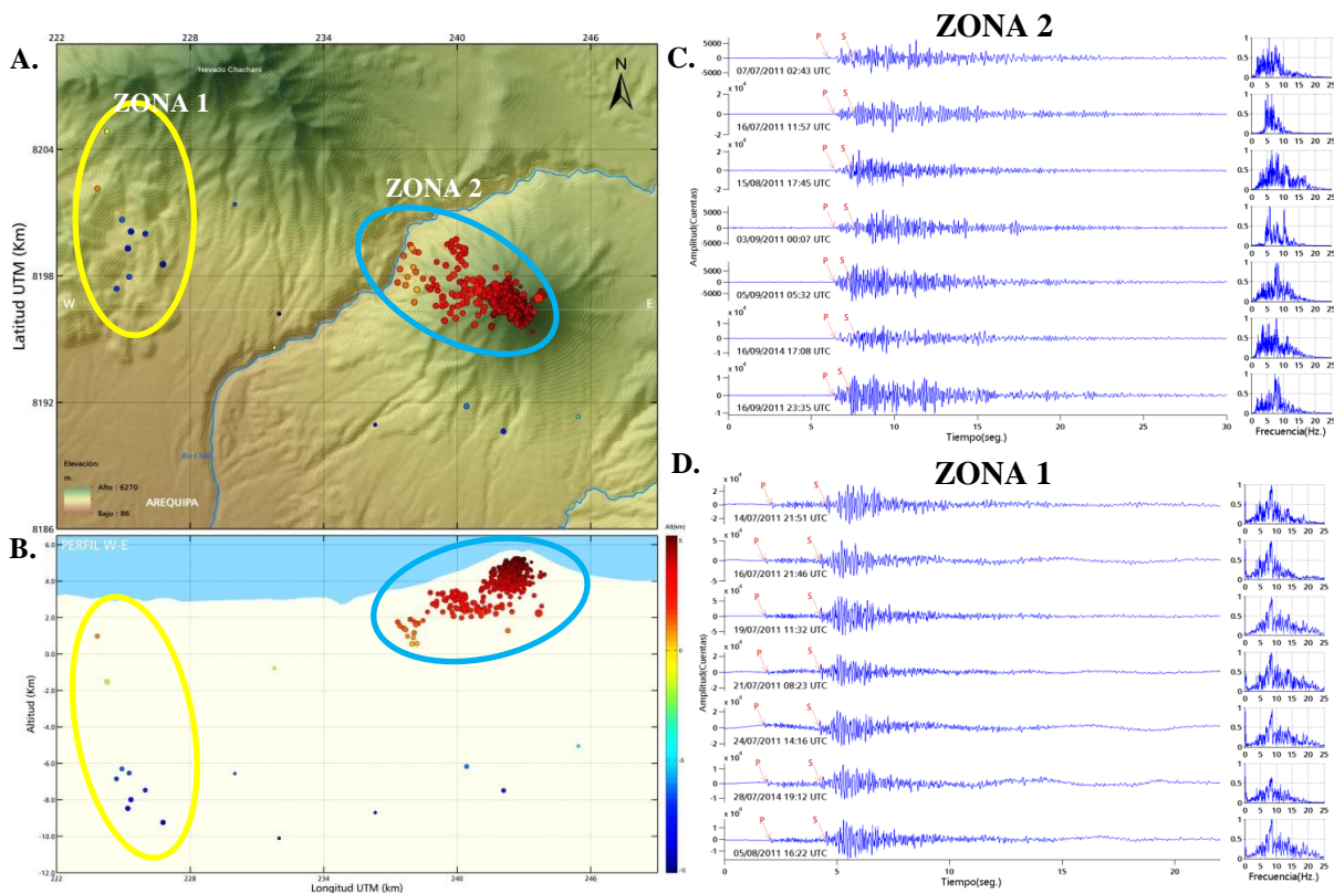
Figura 3.-A) Mapa de distribución epicentral de las dos zonas sismogénicas: Zona 1 y 2, de la región del volcán Misti, B) Corte transversal EW de la sismicidad de la zona de estudio, C) Sismos representativos de la zona 2 y D) Sismos representativos de la zona 1, registrados en la componente vertical de la estación M23, cada uno con su respectivo espectro de frecuencias.
