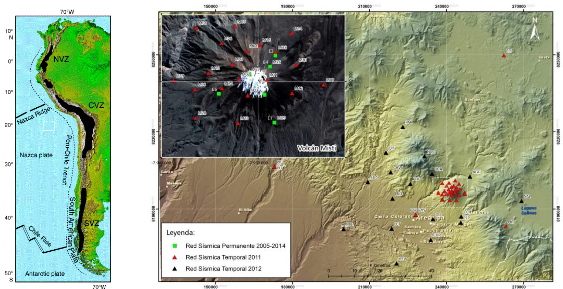
Figura 1.- Mapa de localización de las Estaciones de la campaña sísmica de 2011 y 2012. En el recuadro de la izquierda se observa la ubicación del volcán Misti dentro de la Zona Volcánica Central (CVZ) de América del Sur.
