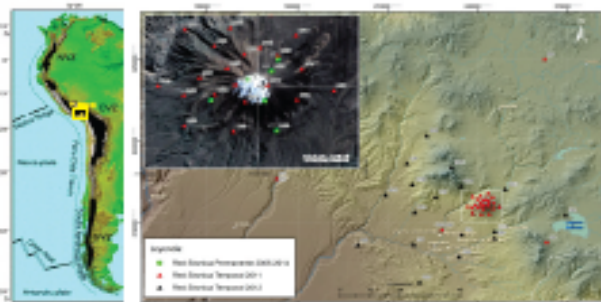
Figura 1.- Mapa de localización de las 5 estaciones sísmicas de la zona volcánica de los volcanes Misti y Chachani en el momento de la configuración de 2005 y 2012. Se ve el estado de las estaciones sísmicas en el momento de la configuración de 2005 y 2012. Se ve el estado de las estaciones sísmicas en el momento de la configuración de 2005 y 2012.
