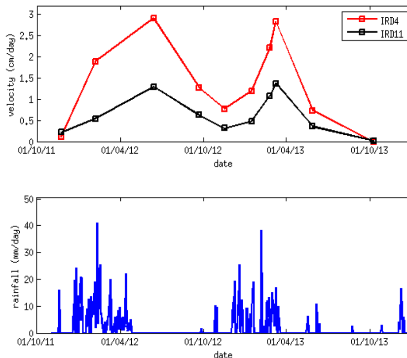
Figura 3. Serie temporal de velocidades de 2 puntos GPS (arriba) y lluvia registrada a la estación meteorológica de Madrigal (abajo).
