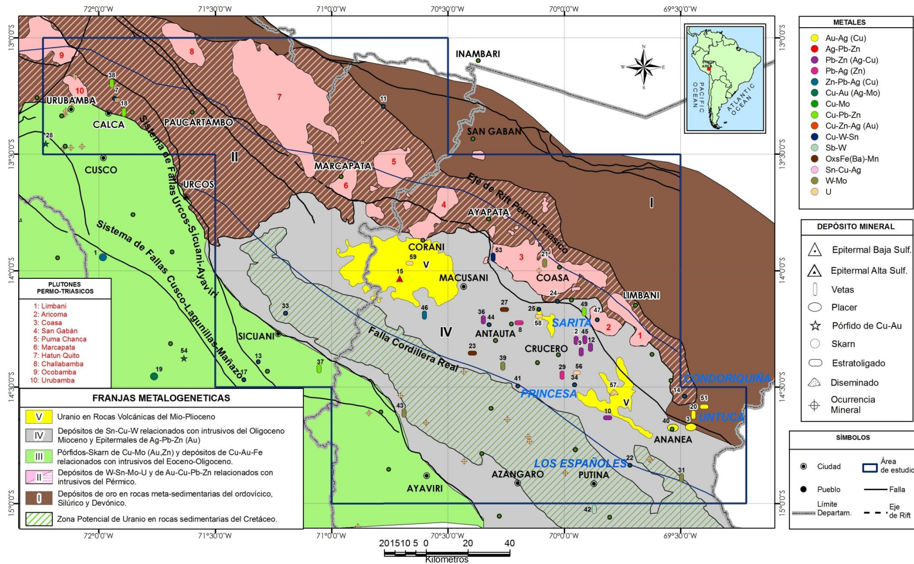
Figura 1.- Franjas metalogénicas y depósitos minerales (ver tabla 3) del área de estudio. Se destacan los intrusivos muestreados y los principales depósitos (en azul) en donde se ha recolectado muestras isotópicas.
