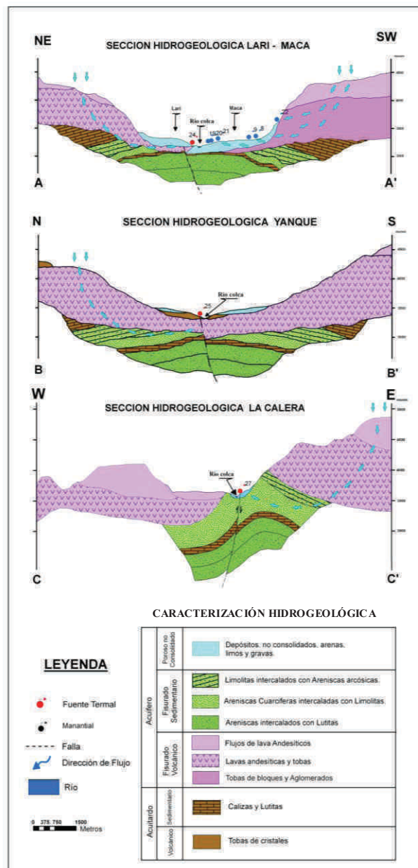
Figura 1. Secciones hidrogeológicas transversales al valle del Colca.
