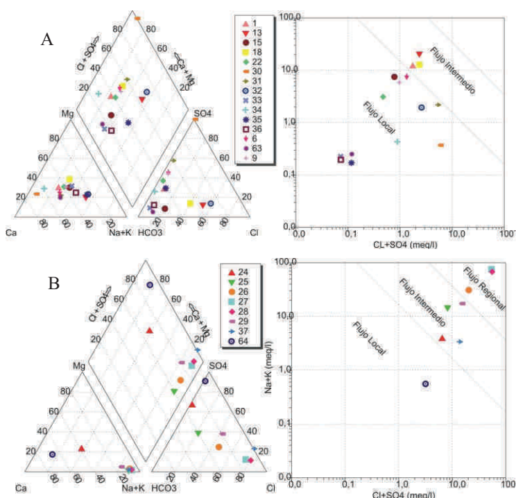
Gráficos 1. A) Diagrama Piper y Scatter para fuentes de aguas frías. B) Diagramas Piper y Scatter para fuentes termales.
