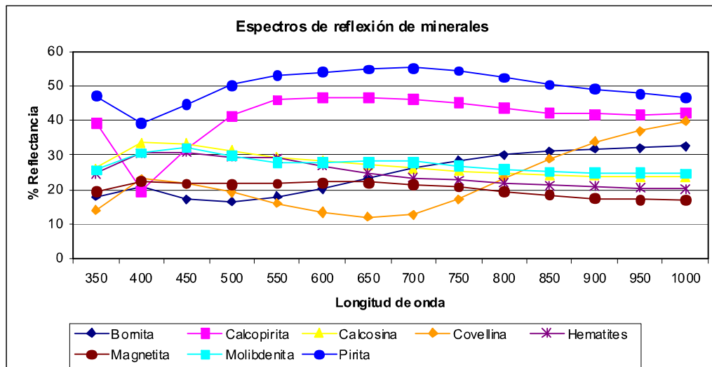
Figura 4: Espectros de reflexión de los minerales estudiados.
