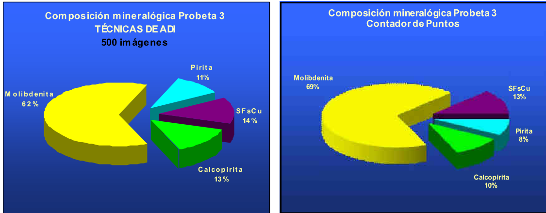
Figura 2: Cuantificación mineral: ADI vs. Contador de Puntos
