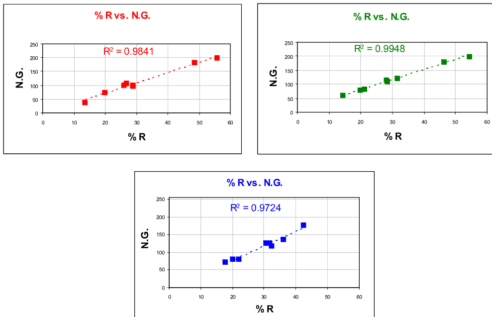
Figura 1: Relación lineal % Reflectancia vs. Niveles de gris.
