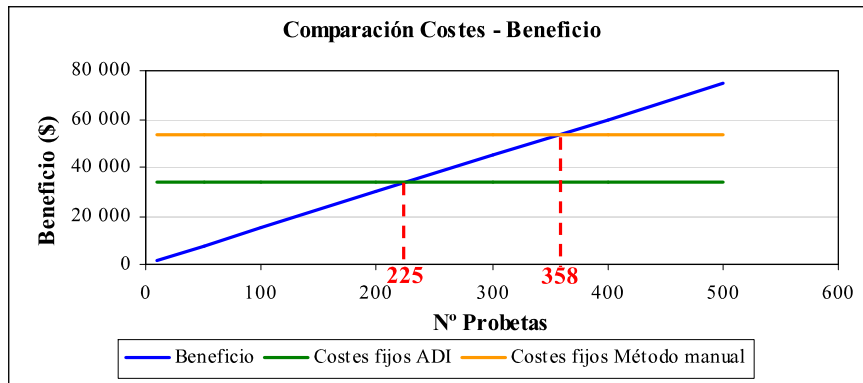
Figura 3: Comparación Costes – Beneficio Método manual vs. ADI.
