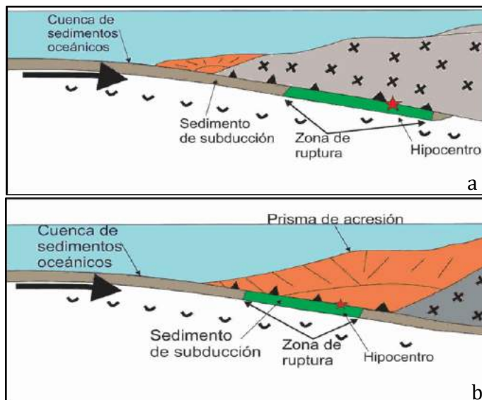
Figura 1: a) Sismos asociados al contacto de placas. b) Sismos asociados al prisma de acreción (Modificado de Kanamori et al., 1993).
