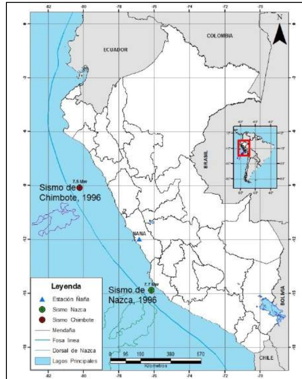
Figura 3: Ubicación de los sismos de Chimbote y Nazca de 1996, así como la estación de Ñaña.
