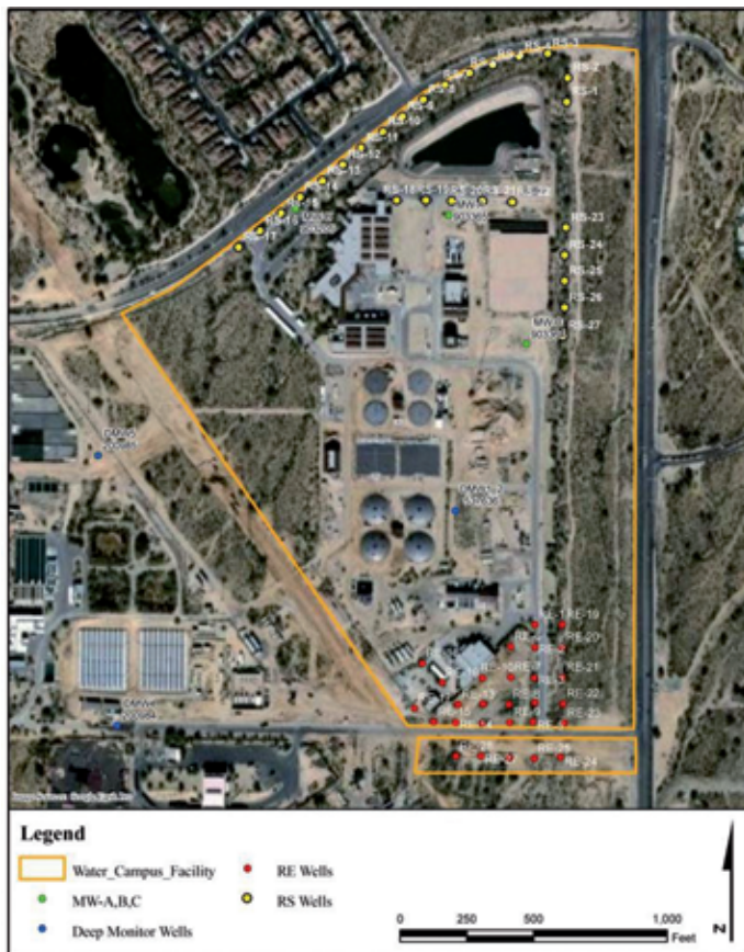
Figure 3. The city of Scottsdale Water Campus facility. A water reclamation and potable water treatment plant performing aquifer storage using vadose zone recharge wells and ASR wells Figura 3. La instalación del Campus del Agua en la ciudad de Scottsdale. Es una planta depuradora y potabilizadora que posibilita el almacenamiento en el acuífero mediante pozos de recarga en la zona no saturada y pozos ASR
