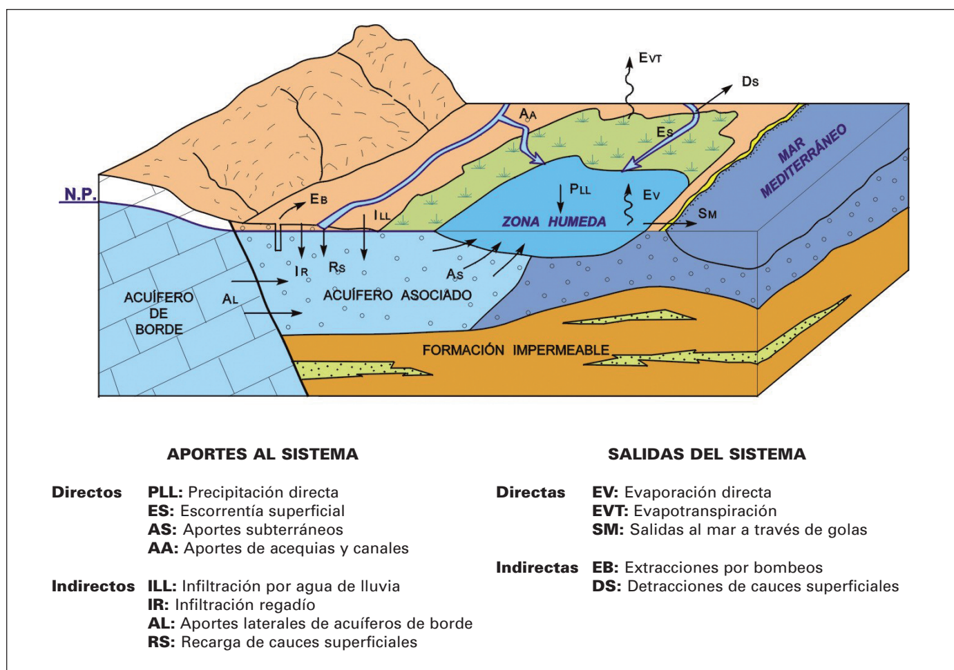
Figura 1. Elementos que integran el balance hídrico de un humedal litoral mediterráneo (Ballesteros, 2003)
