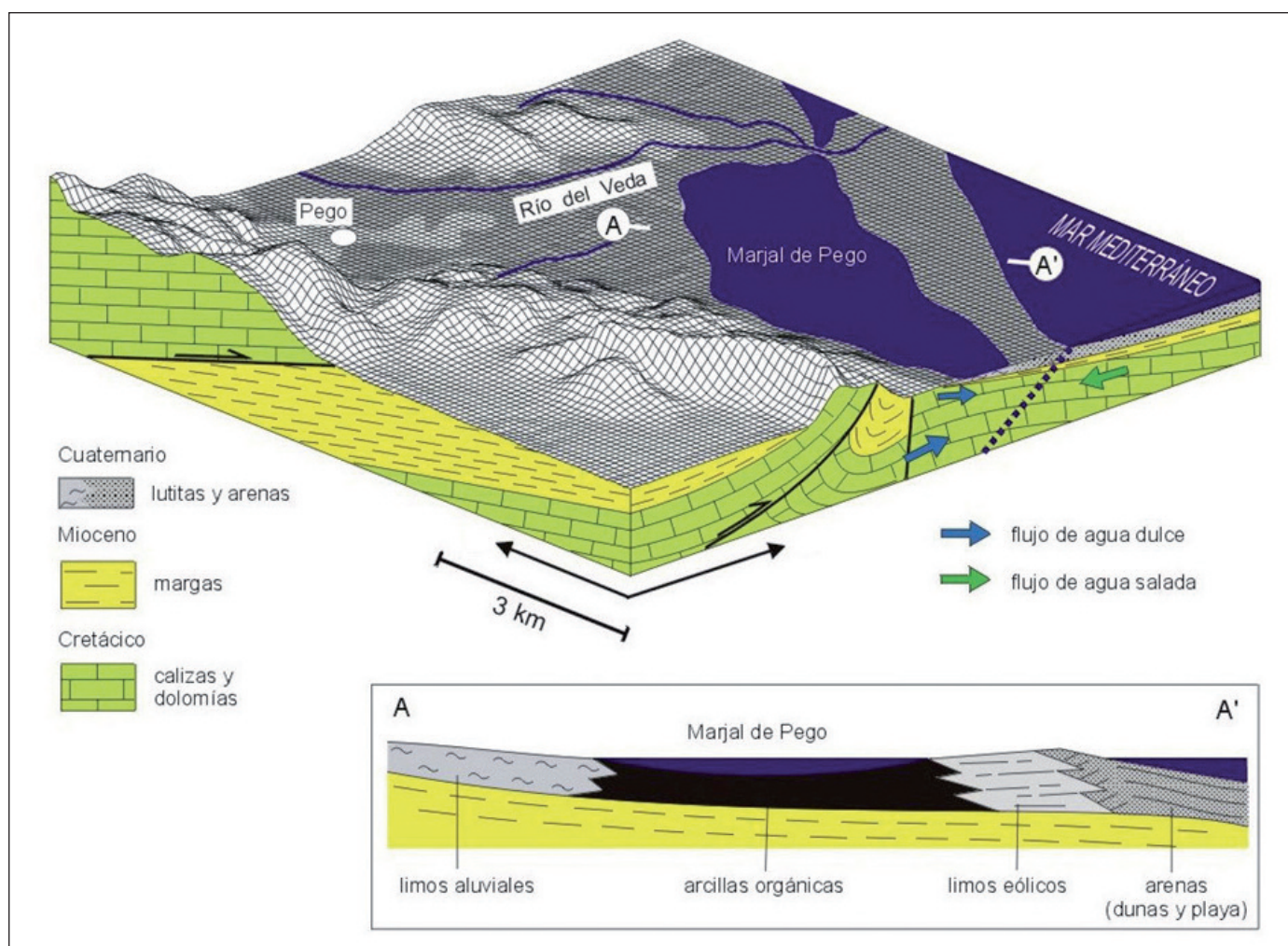
Figura 5. Modelo geológico de la marjal de Pego-Oliva (Durán et al., 2005)
