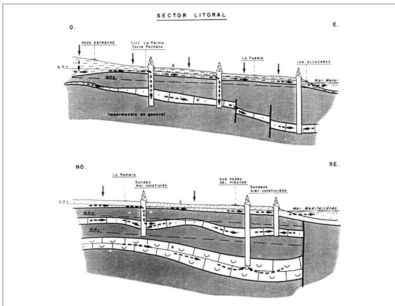
Figura 7. Sección representativa del sector litoral del Campo de Cartagena (ITGE, 1992)
