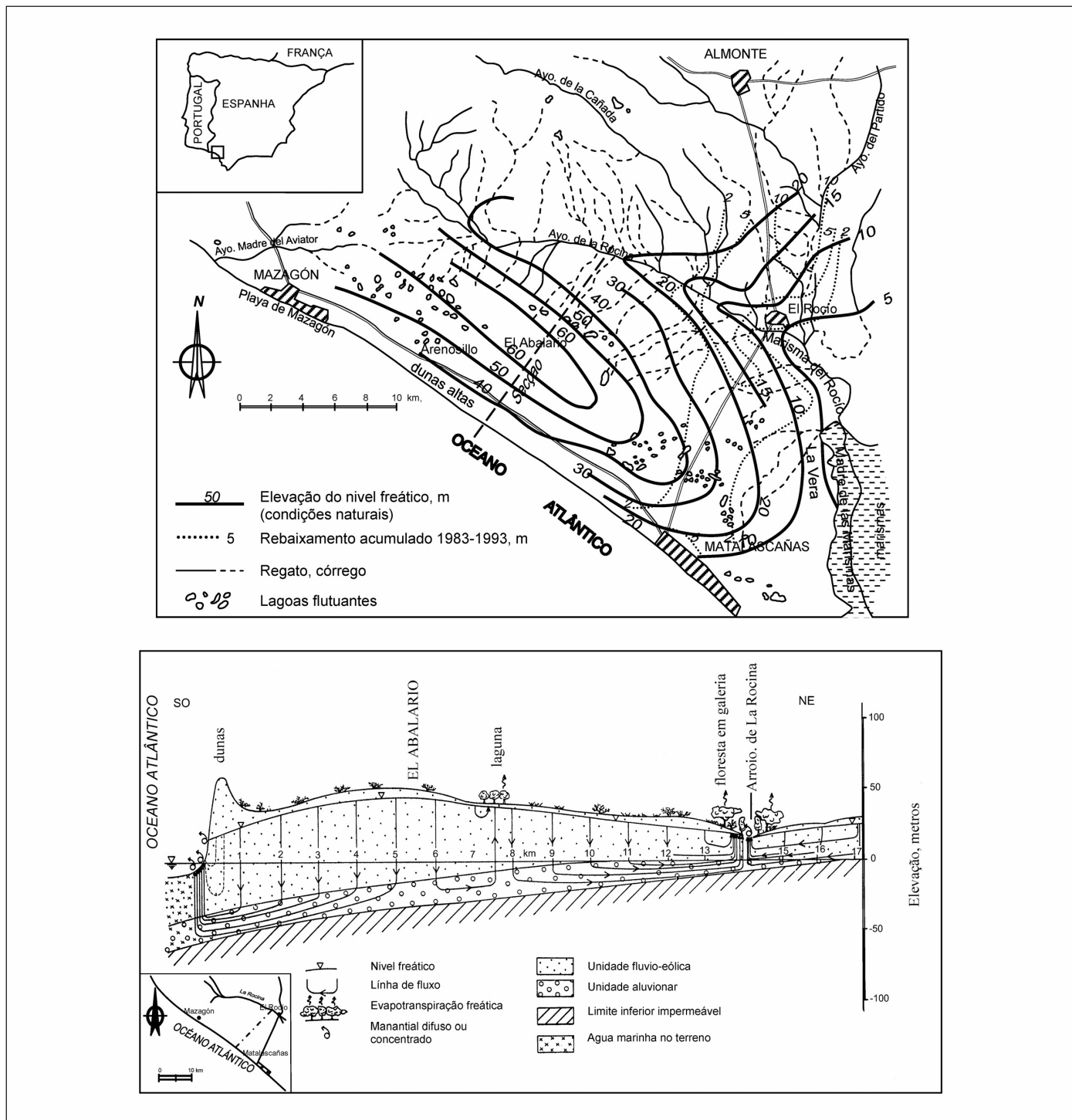
Fig. 2. Padrão de fluxo tridimensional de águas subterrâneas idealizado em uma seção através da formação arenosa de El Abalarío (Doñana, Sul da Espanha) onde um aquífero profundo ocorre sob uma potente camada de areias siliciclásticas finas a médias e que contém o aquífero livre. A água subterrânea fluindo através da areias é descarregada em fontes e como fluxo difuso na linha de costa e no riacho La Rocina, bem como pelas plantas próximo a La Rocina e em áreas intermediárias de aquíferos freáticos rasos. A presença de formações de baixa permeabilidade tem grande influência no padrão de fluxo local (modificado de Custodio e Palancar, 1995; Custodio, 1995) Fig. 2. Idealized three-dimensional flow pattern in a cross-section through the El Abalarío sandy formation (Doñana, southern Spain) where a deep aquifer underlies a thick layer of fine to medium silica sands containing the water-table. Groundwater flowing through the sands outflows in springs and as diffuse flow at the coast line and at the La Rocina ravine, as well as through the plants near La Rocina and in intermediate areas with shallow water-table. The existence of low permeability formations has a great influence in the local flow pattern (modified from Custodio and Palancar 1995; Custodio 1995)
