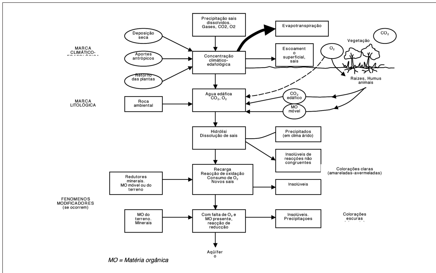
Fig. 1. Representação simplificada e idealizada de como a composição química da água subterrânea é gerada. A figura refere-se à recarga difusa por precipitação (modificado de Candela et al. , 1998)
