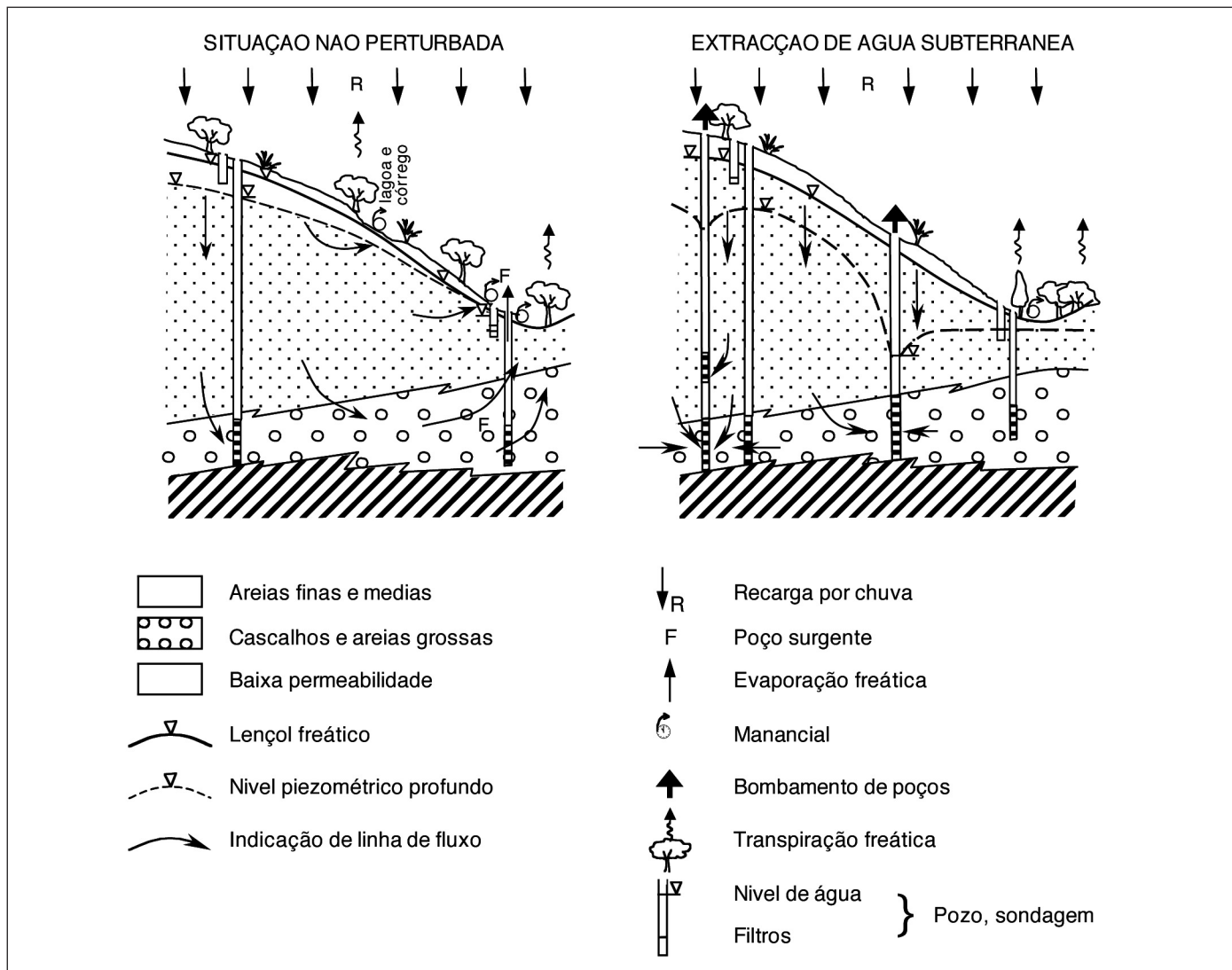
Fig. 4. Esquema idealizado das relações entre o nível freático e o nível piezométrico profundo no sistema aquífero de El Abalarío, área de Doñana (Sul de Espanha) de areias finas sobre uma formação profunda grosseira onde estão os filtros dos poços. Situações natural e perturbada por bombeamentos. Põe-se atenção nos efeitos ambientais (mananciais, riacho, lagoas e vegetação)
