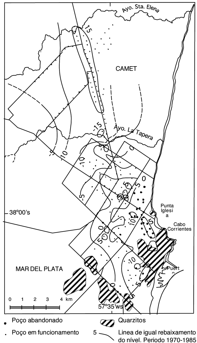
Fig. 7. Resultados da extração de água subterrânea em áreas urbanas e de periferia da cidade de Mar del Plata (Argentina), após parte dos poços da cidade terem sido fechados devido à má qualidade e contaminação salina, e substituídos por poços na periferia. As isolinhas mostram as mudanças no nível freático (em metros) entre 1970 e 1985 (segundo Bocanegra et al., 1992). Enquanto ocorre um progressivo rebaixamento do nível freático na zona periférica, na cidade ocorre uma recuperação que afeta as fundações de alguns edifícios altos devido à subpressão e ao ambiente corrosivo resultante da presença de água salgada
