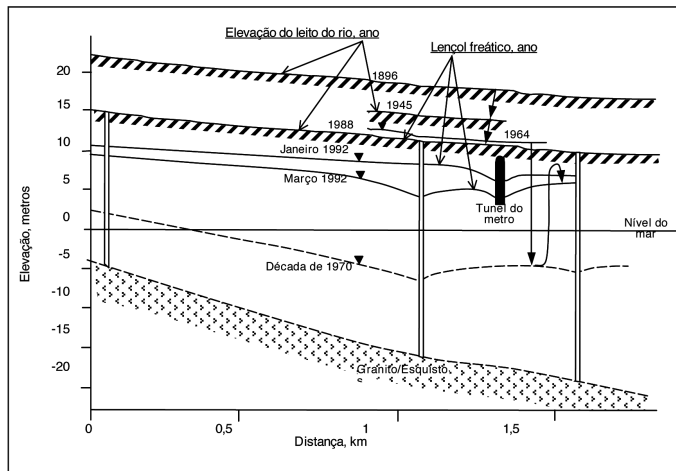
Fig. 6. Áreas ameaçadas de alagamentos e com ocorrência destes no ano de 1982 (segundo Custodio e Bayó, 1986), na planície costeira de Barcelona (figura superior), devido ao abandono progressivo de poços em áreas originalmente correspondentes a aquíferos com nível freático raso. Isso afeta estruturas subterrâneas, tais como a rede de metrô. A figura inferior mostra esse efeito em um trecho sob o rio (Vázquez-Suñé e Sánchez-Vila, 1997; Vázquez-Suñé et al., 1997)
