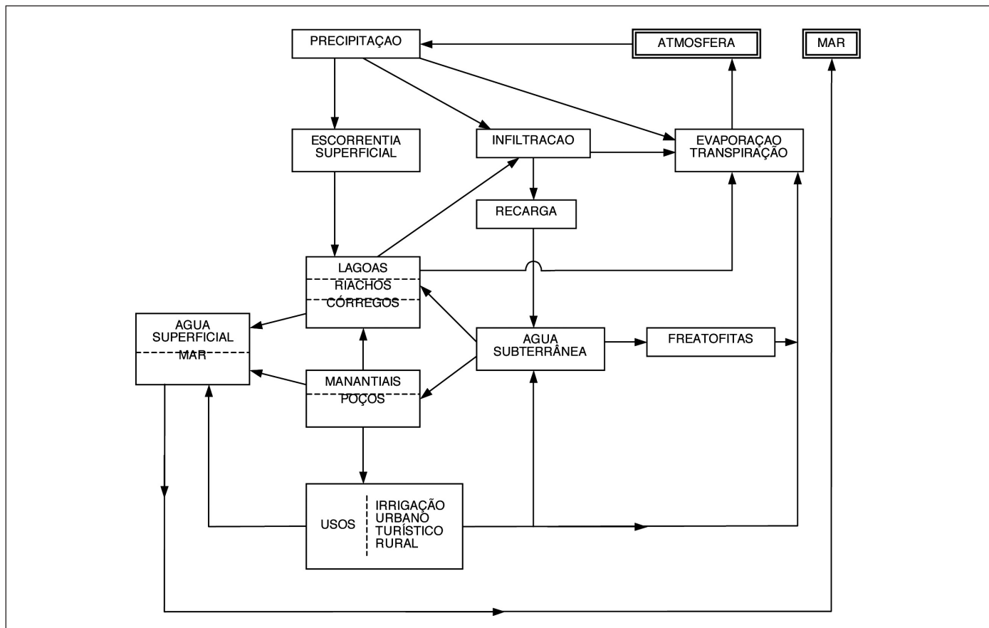
Fig. 3. Diagrama esquemático dos elementos do balanço de água na área de Doñana (Sul de Espanha). Estes diagramas são um resumo do modelo conceitual
