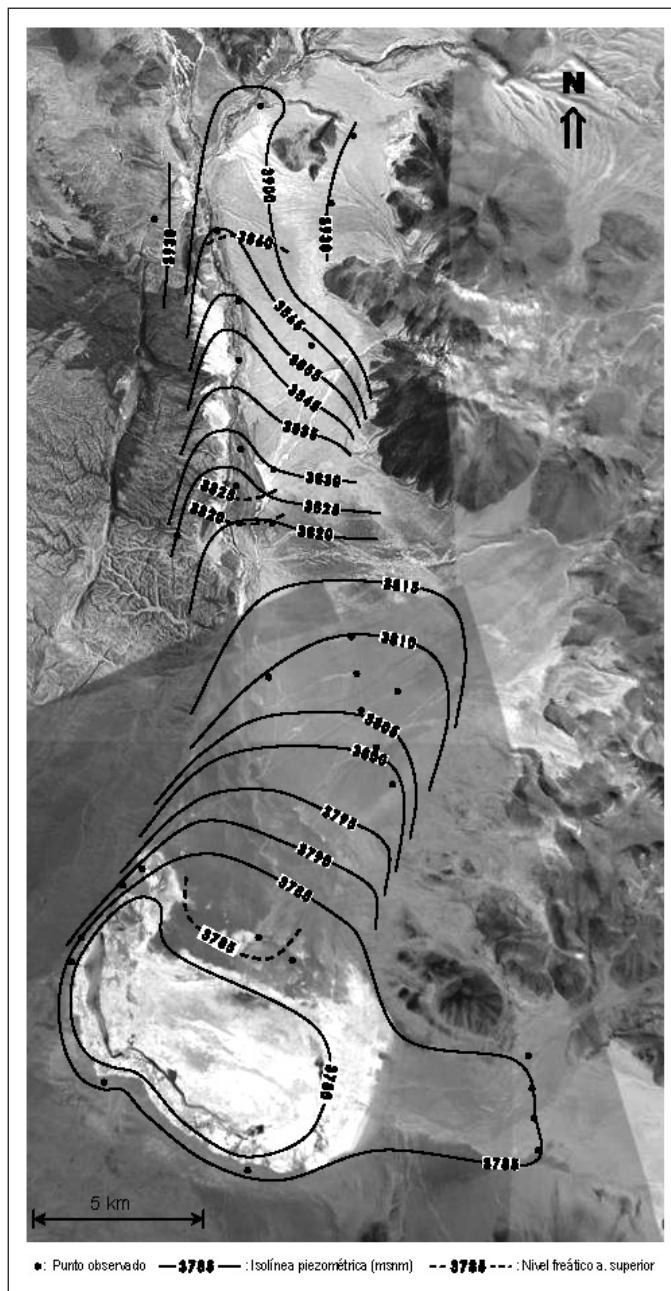
Fig. 7. Piezometría de los acuíferos superior y medio-inferior durante el año 2001, en metros snm
