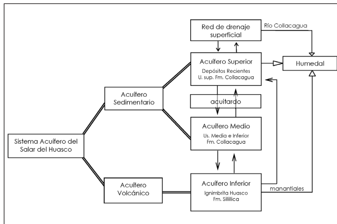
Fig. 11. Esquema simplificado del funcionamiento hídrico del sistema acuífero del Salar del Huasco Fig. 11. Simplified Chart of the functioning of the aquifer system of Salar del Huasco
