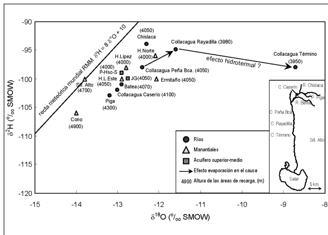
Fig. 10. Valores de \delta^{18}\text{O} y \delta^2\text{H} en las aguas del Salar del Huasco en relación con la recta del agua meteorológica mundial (RMM) que es aproximadamente igual a la local para el norte de Chile
