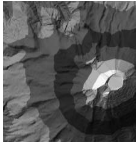
Fig. 10. Modelo digital de elevación del volcán Popocatepetl
