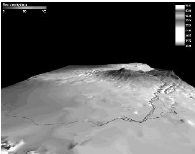
Fig. 9. Modelo tridimensional del volcán Popocatepetl.
