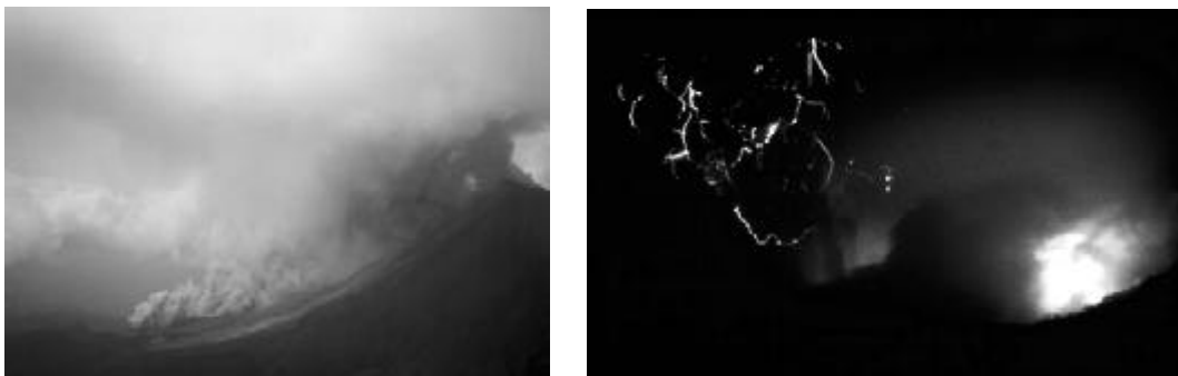
Fig. 21. Izquierda: Flujo piroclástico de magnitud moderada producido por el derrumbe de bloques de lava en el volcán de Colima a finales de 1998. Numerosos flujos de este tipo han motivado varias evacuaciones preventivas de poblaciones cercanas a ese volcán. Derecha: Flujo piroclásticos de gran tamaño y poder destructivo, generado durante la erupción del volcán El Chichón, el 3 de abril de 1982. Fotografías de S. De la Cruz.
