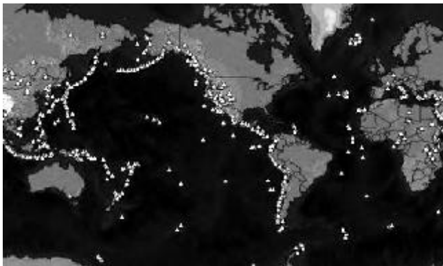
Fig. 5. Distribución geográfica de volcanes en el mundo.
